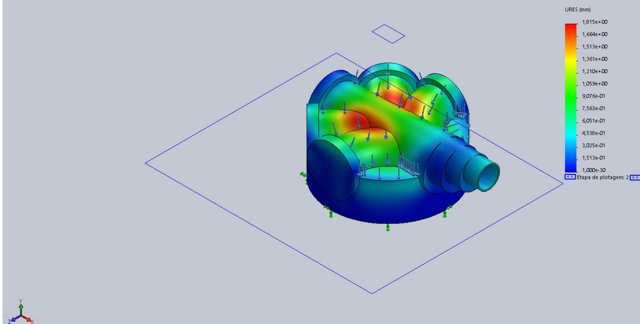
PV 1000 Ensaio Fundo-Não linear 1-Deslocamento-Deslocamento1
